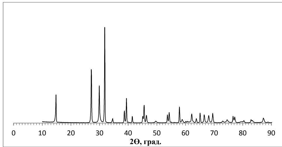
Рис.8. Дифрактограмма (CoK \alpha ) MoO 3 (№ 8, Таблица № 6)
