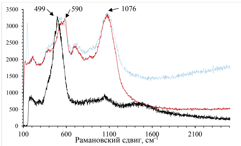
Рис. 128. КРС спектры композита графен-NiO, снятые в разных точках, при возбуждении лазером с длиной волны 514 нм.
