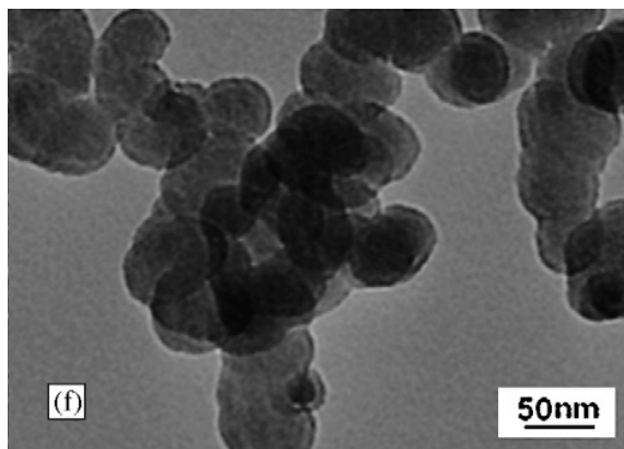
Рис. 6. Микрофотография, полученная с помощью ПЭМ, порошка \text{Co}_3\text{O}_4 , синтезированного сольвотермальным методом [72].
