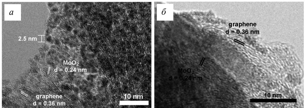
Рис. 43. Микрофотографии (ПЭМВР) композита ВОГ- \text{MoO}_2 , синтезированного методом восстановления [162].
