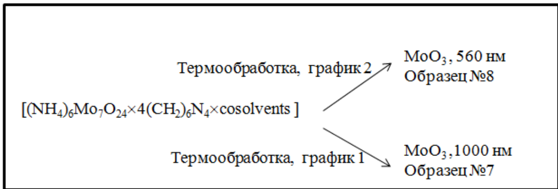
Схема 1. Влияние режима термообработки геля при исходном мольном отношении GMTA/Mo 7 , равном 4, на дисперсность прокаленных порошков MoO 3 (образцы 7 и 8 в Таблице 6).
