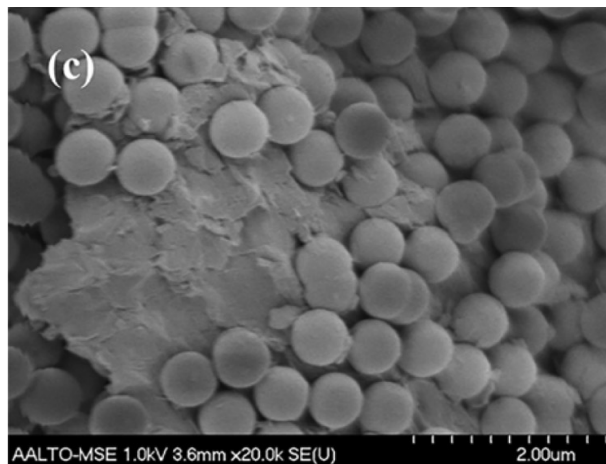
Рис. 48. Микрофотография, полученная с помощью СЭМ, композита ВОГ-SiO 2 , синтезированного гидротермальным методом [167].
