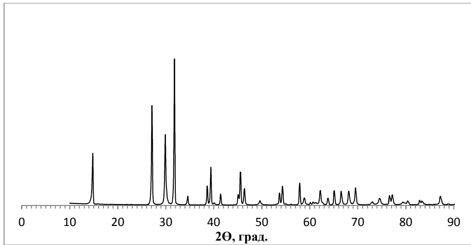
Рис.7. Дифрактограмма (CoK \alpha ) MoO 3 (№ 7, Таблица № 6)
