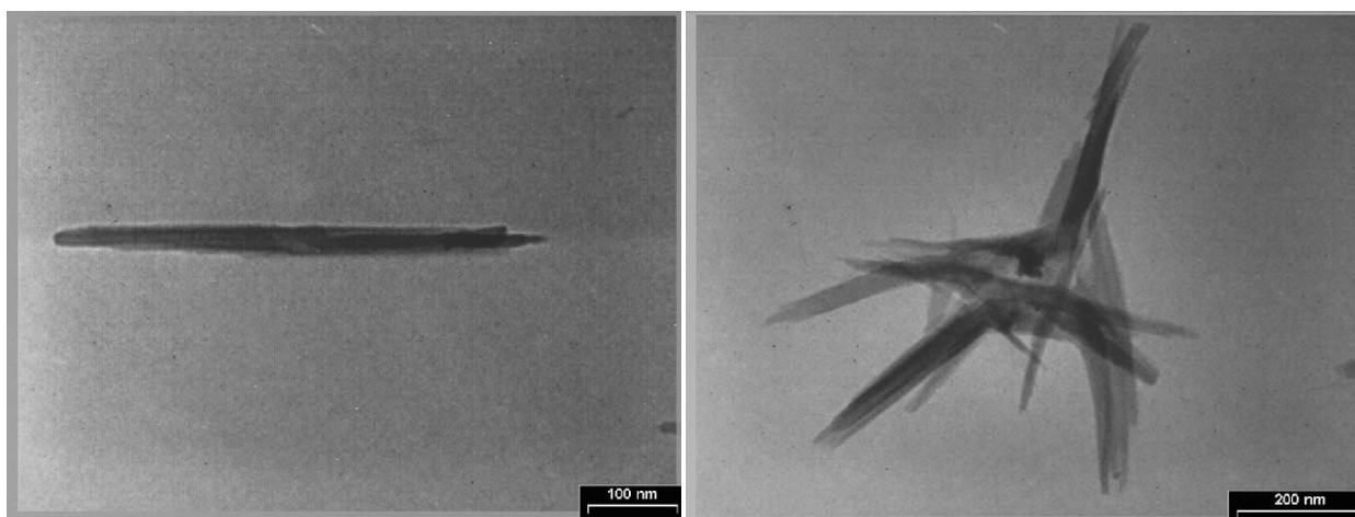
Рис. 1. Микрофотографии, полученные с помощью ПЭМ, стержней \text{Co}_3\text{O}_4 , синтезированных термическим разложением оксалата кобальта [68].
