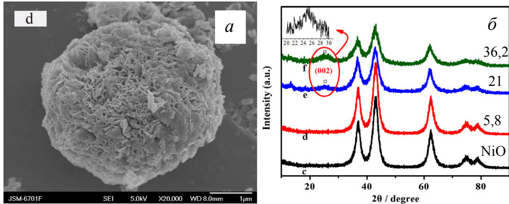
Рис. 37. Микрофотография (СЭМ) (а) и дифрактограммы (б) композитов ВОГ-NiO, синтезированных сольвотермальным методом [155].
