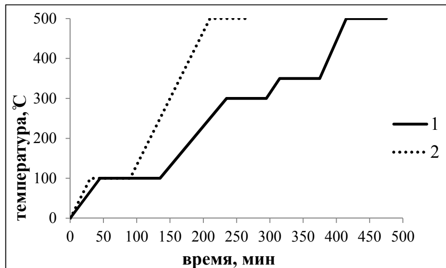
Рис. 58. Используемые графики повышения температуры при термообработке синтезированных золь-гелей.
