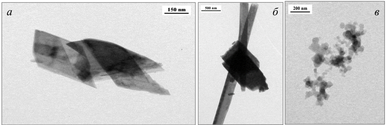
Рис. 60. Полученные с помощью ПЭМ микрофотографии порошка \text{MoO}_3 , синтезированного с использованием ГМТА (образец 3 в Таблице 6).
