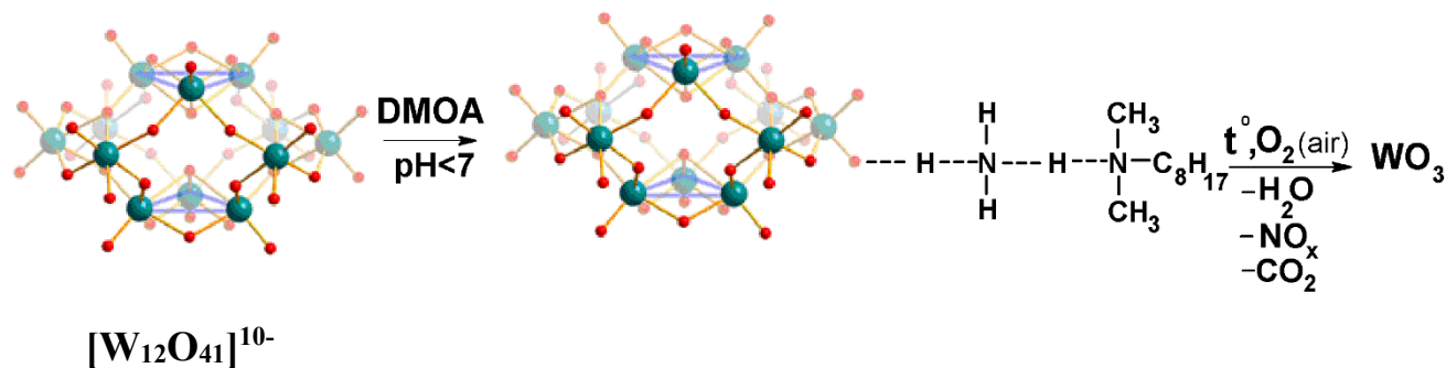
Схема 5. Предполагаемый механизм формирования наночастиц WO_3 .
