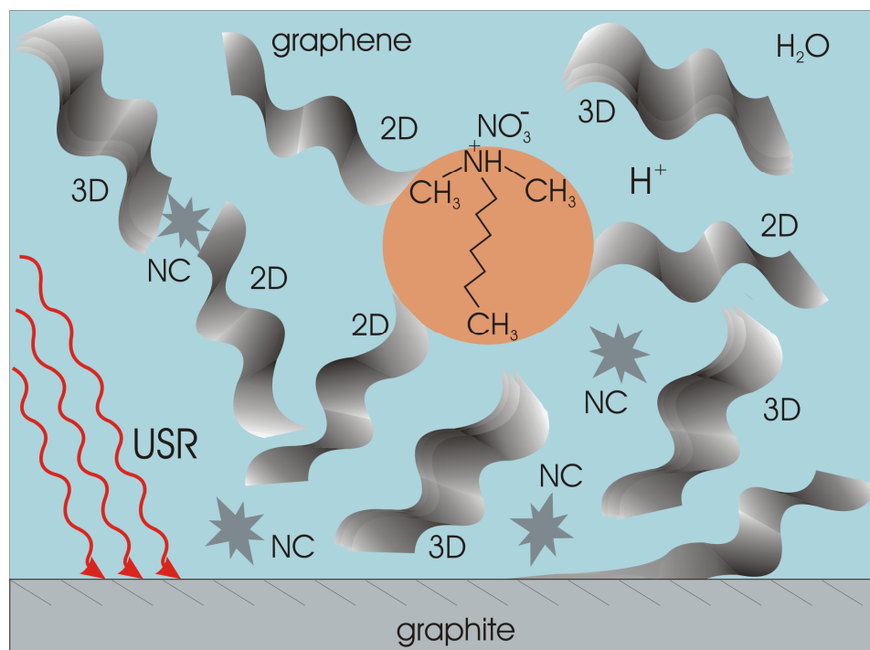
Рис. 89. Схема образования графеновых листов из графита в эмульсии, содержащей микрокапли N,N-диметилноктиламина.
