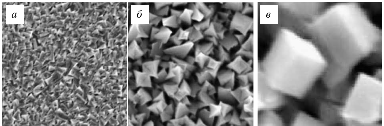
Рис. 9. Микрофотографии (СЭМ) пленок шпинели \text{Co}_3\text{O}_4 , осажденных при 360°C ( a ), 430°C ( б ), 540°C ( в ) [74].
