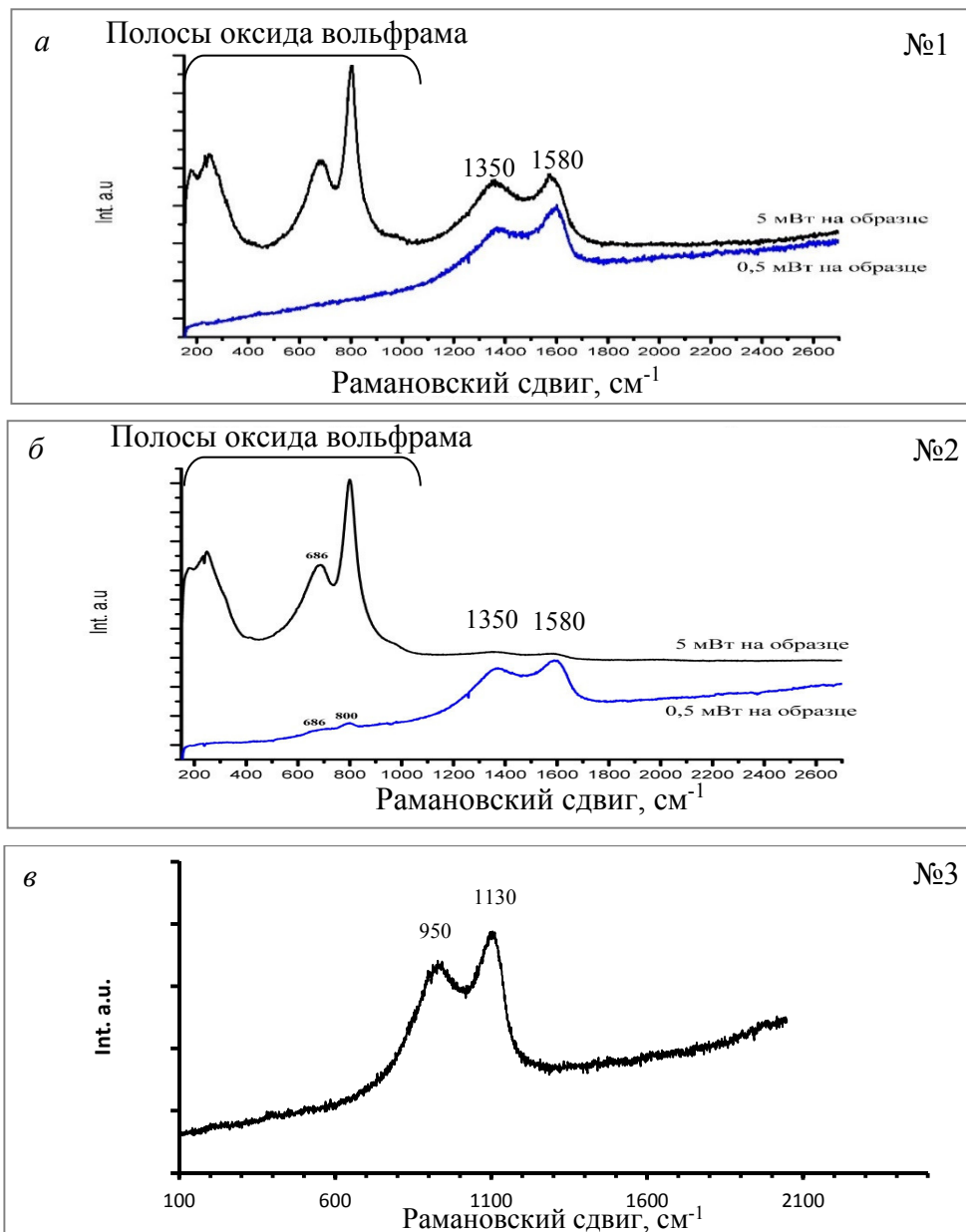
Рис. 116. КРС спектры композитов графен- \text{WO}_3 №№1-3 (нумерация Таблицы 14) при возбуждении лазером с длиной волны 514 нм.
