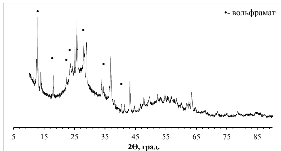
Рис. 120. Дифрактограмма ( \text{CuK}\alpha ) композита графен- \text{WO}_3 (образец 4, Таблица 14).
