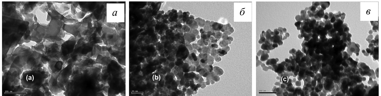
Рис. 8. Микрофотографии (ПЭМ) порошков \text{Co}_3\text{O}_4 , синтезированных гидротермальным методом с использованием в качестве источника металла \text{CoSO}_4 ( a ), \text{CoCl}_2 ( б ), \text{Co}(\text{NO}_3)_2 ( в ) [73].
