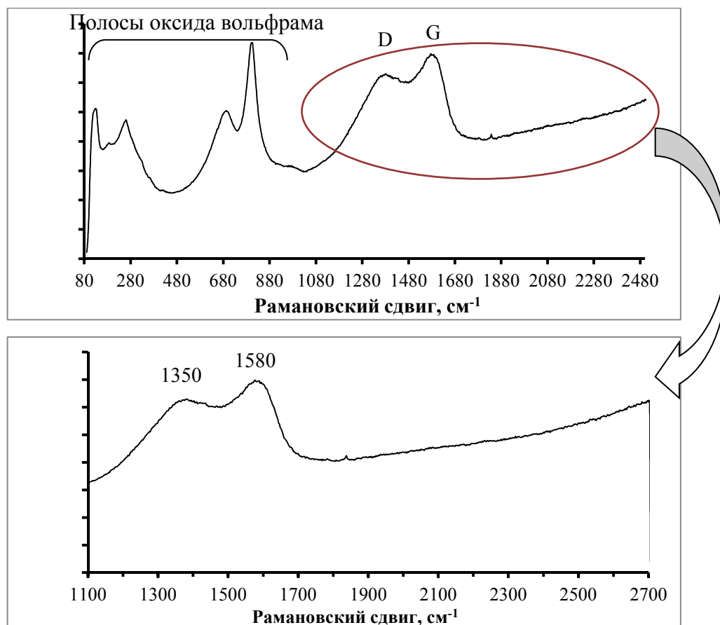
Рис. 119. КРС-спектр композита графен- WO_3 , синтезированного с использованием графеновой суспензии, полученной при продолжительности ультразвуковой эксфолиации, равной 15 мин. (образец 4, Таблица 14).
