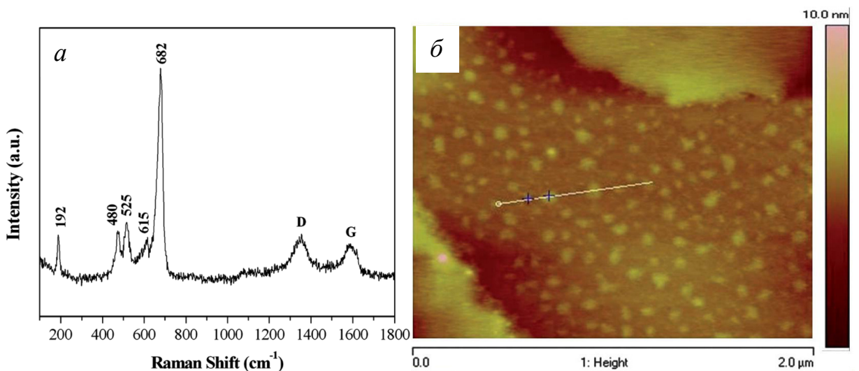
Рис. 31. КРС-спектр (а) и микрофотография (б), полученная с помощью АСМ, композита графен- \text{Co}_3\text{O}_4 , синтезированного методом химического восстановления [150].
