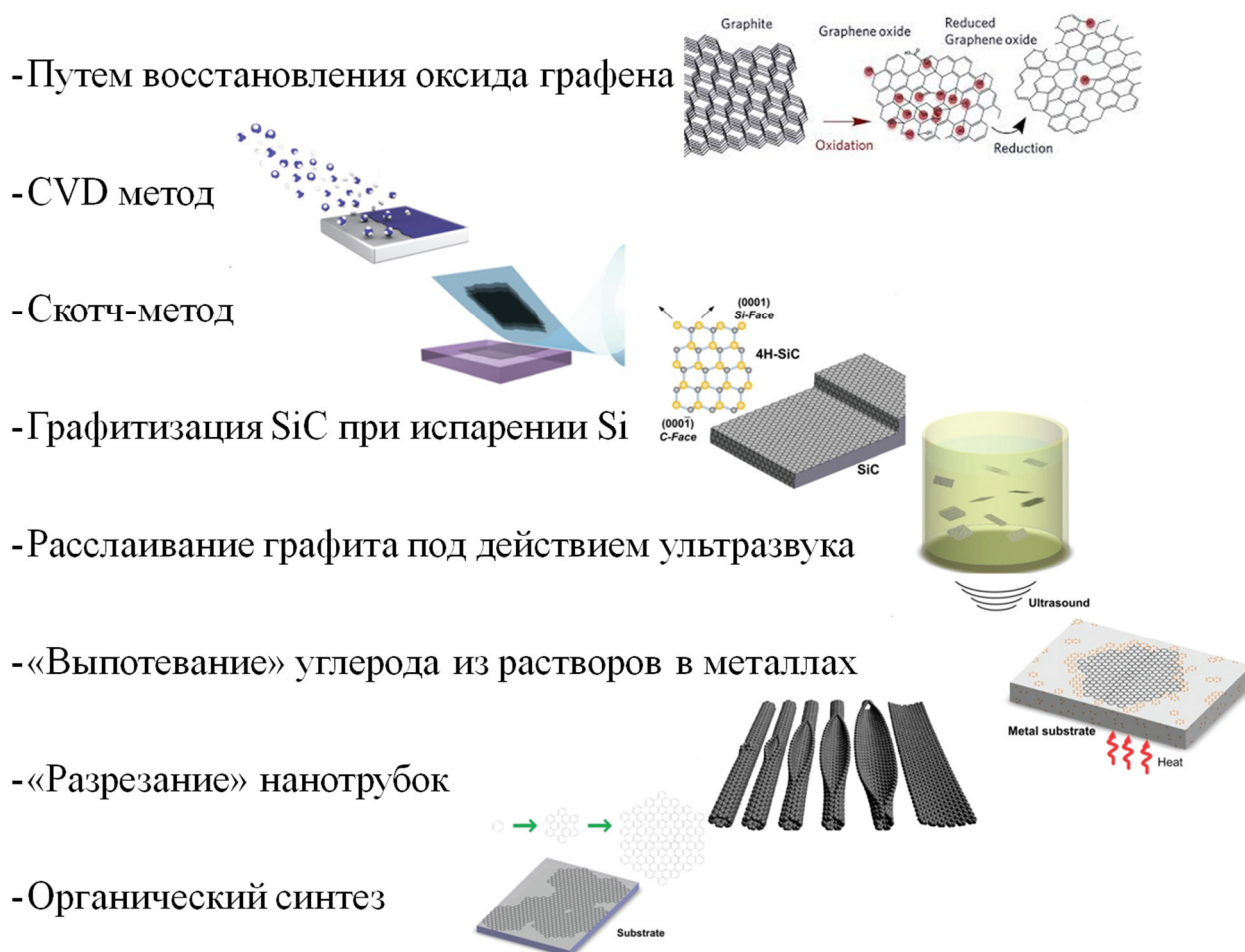
Рис. 29. Методы получения графеновых структур
