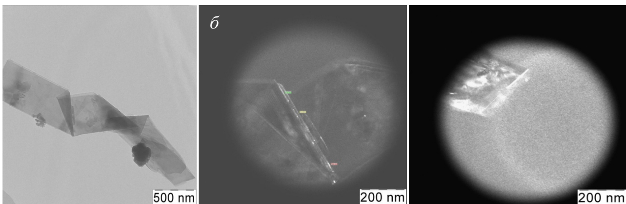
Рис. 94. Микрофотографии, полученные с помощью ПЭМ, графеновых лент при обычной съемке (а) и в темнопольном режиме (б и в).
