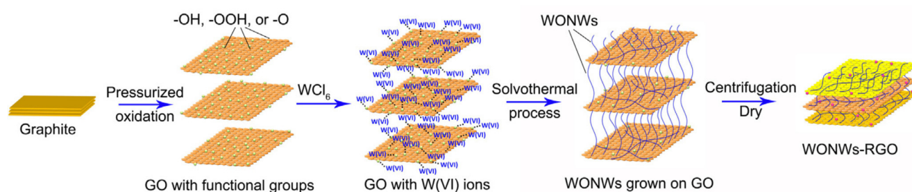
Рис. 44. Схема образования «сэндвичевых» структур при использовании сольвоотермального метода [163].
