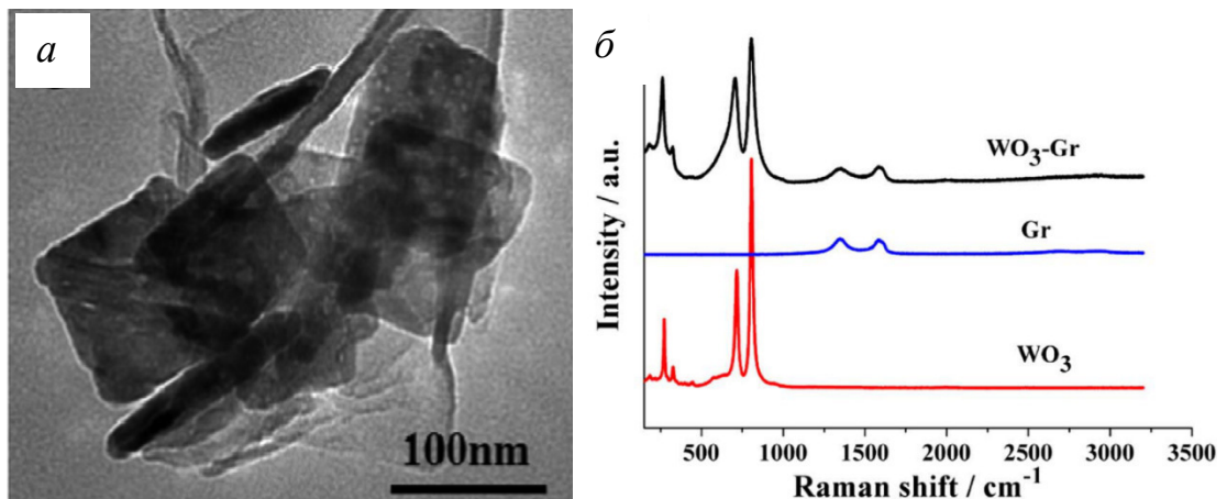
Рис. 46. Микрофотография, полученная с помощью ПЭМ (а), и КРС-спектры композита \text{VOG-WO}_3 , синтезированного гидротермальным методом (б) [165].
