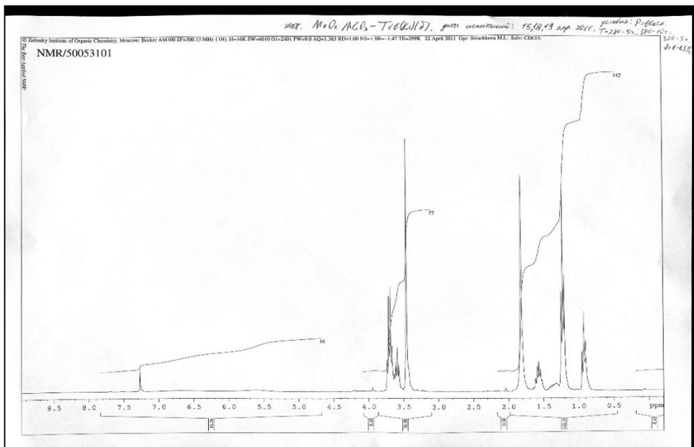
Рис. 3. Результат исследования методом ^1\text{H} ЯМР жидких продуктов, полученных на катализаторе \text{K1}_s .
