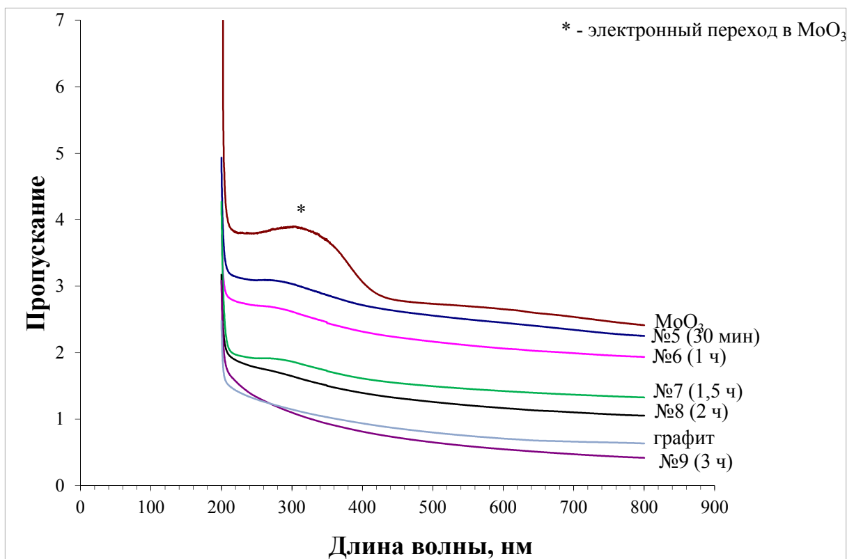
Рис. 114. УФ-спектры композитов графен-МоО 3 , синтезированных с использованием суспензий графена, полученных при различной продолжительности ультразвукового воздействия на графит (образцы №№ 5-9, Таблица 13).
