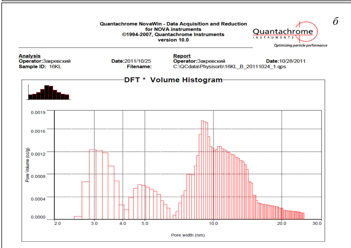
Рис. 6. Результаты адсорбции-десорбции N_2 на катализаторе K1: a – синяя кривая распределения по размеру (диаметру) пор, красная кривая полного объема пор, б – гистограмма распределения по объему пор.
