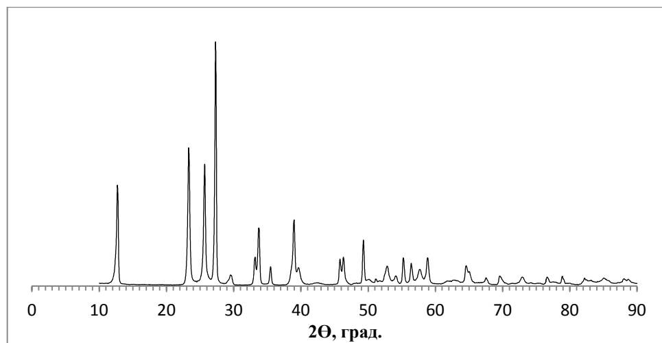
Рис.9. Дифрактограмма (CuK \alpha ) MoO 3 (№ 9, Таблица № 6)
