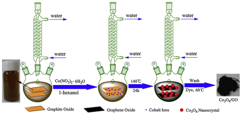
Рис. 32. Схема получения композита ОГ- \text{Co}_3\text{O}_4 сольвотермальным методом [151].
