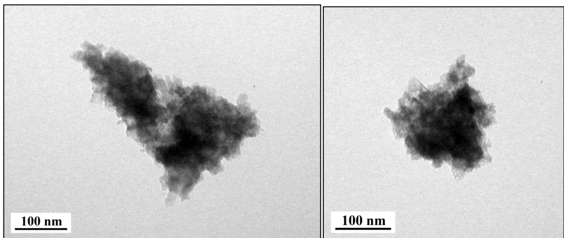
Рис. 4. Микрофотографии катализатора К1, полученные с помощью ПЭМ.
