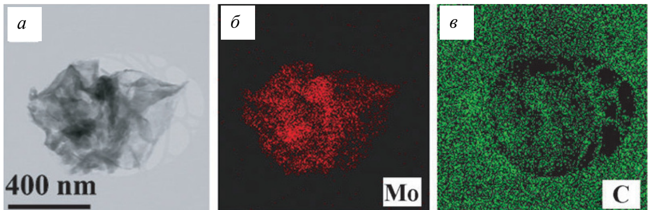
Рис. 42. Микрофотография, полученная с помощью ПЭМ, композита ВОГ- \text{MoO}_3 (а), распределение Mo (б) и C (в) в композите [161].
