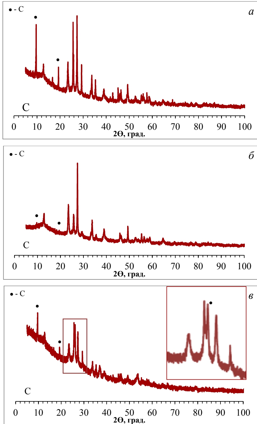
Рис. 107. Дифрактограммы ( \text{CuK}\alpha ) синтезированных композитов графен- \text{MoO}_3 при отношении ДМОА/С (графит) в реакционной среде 0,5 ( a ), 1 ( b ), 1,5 ( в ).
