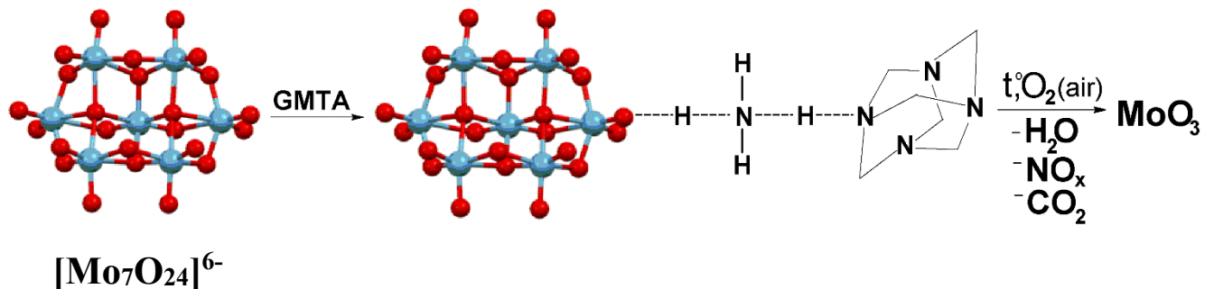
Схема 3. Предполагаемый механизм формирования наночастиц \text{MoO}_3 .
