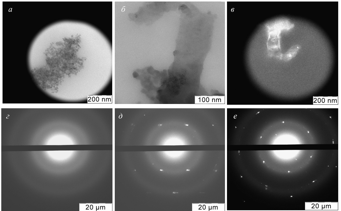
Рис. 132. Микрофотографии, полученные с помощью ПЭМ, нанопорошка \text{SiO}_2 ( a ), гибридных наноструктур графен- \text{SiO}_2 в светлом ( б ) и темном поле ( в ) и дифракция электронов на них ( г , д , е , соответственно).
