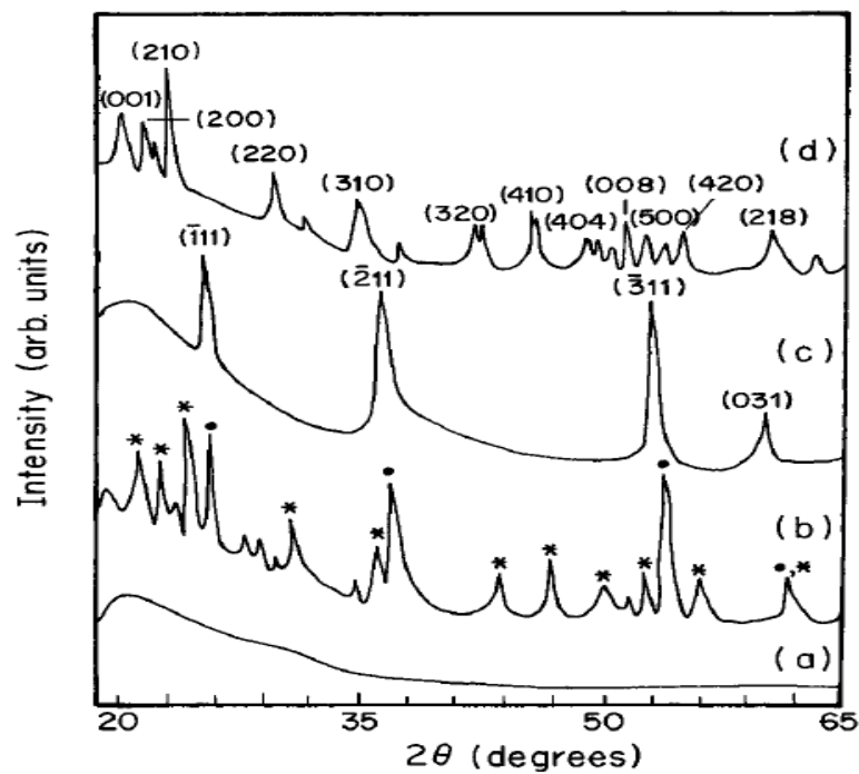
Рис. 23. Дифрактограммы порошка оксида молибдена, синтезированного с помощью приемов сонохимии (а) и прокаленного в атмосфере азота (б), водорода (с), кислорода (д) [89].
