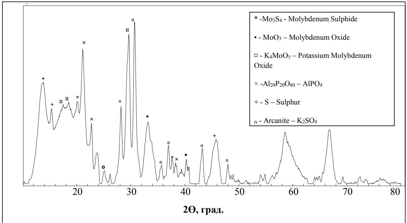
Рис. 1. Дифрактограмма сульфидированного катализатора K1 s .
