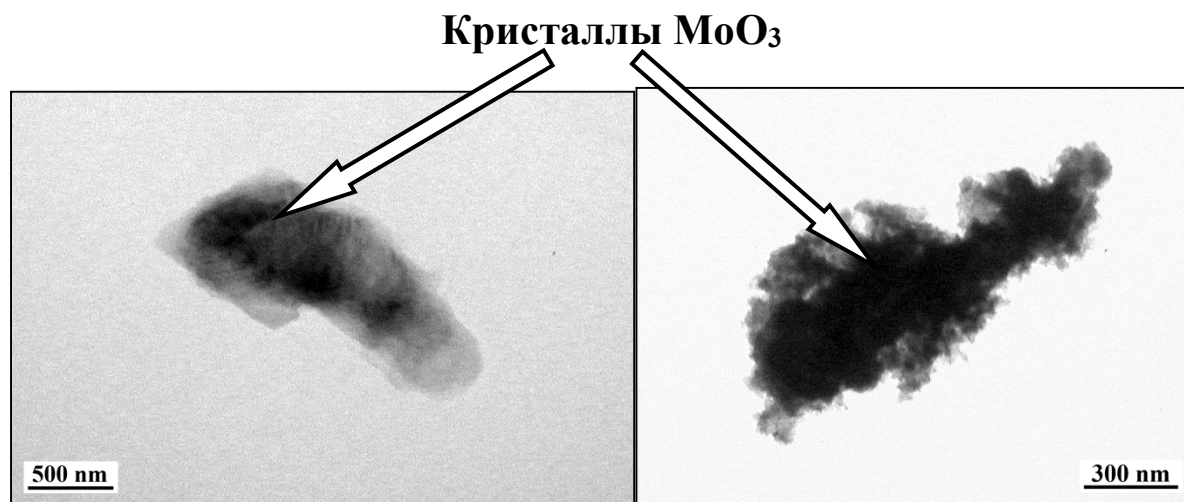
Рис. 8. Микрофотографии катализатора K2, полученные с помощью ПЭМ.
