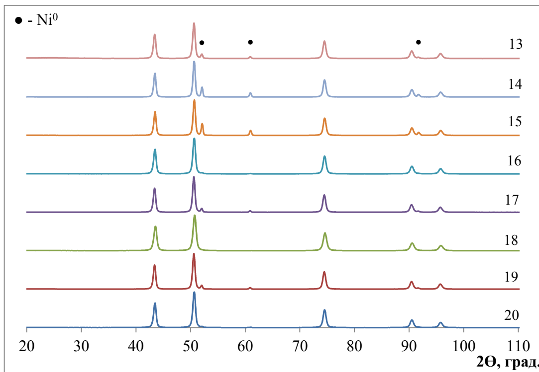
Рис. 81. Дифрактограммы порошков NiO, полученных с использованием АсАс в качестве комплексообразователя (нумерация Таблицы 10). Дифрактограммы сняты с использованием CoK_{\alpha} -излучения.
