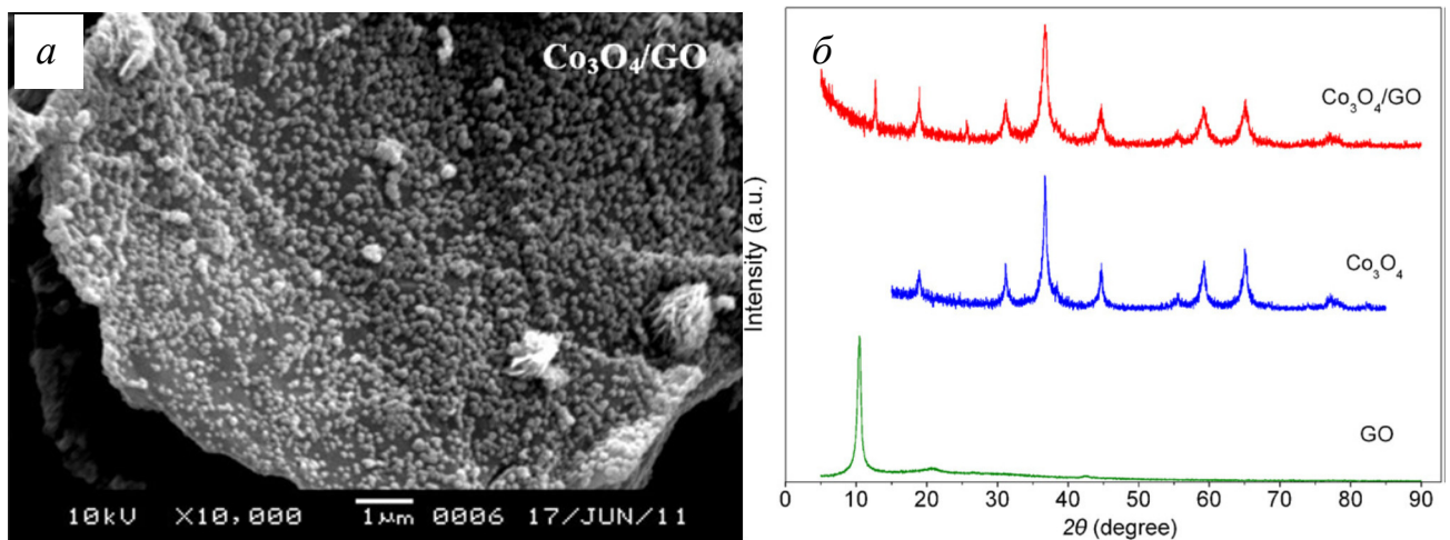
Рис. 33. Микрофотография, полученная с помощью СЭМ (а), и дифрактограмма (б) композита ОГ- \text{Co}_3\text{O}_4 , синтезированного сольвотермальным методом [151].
