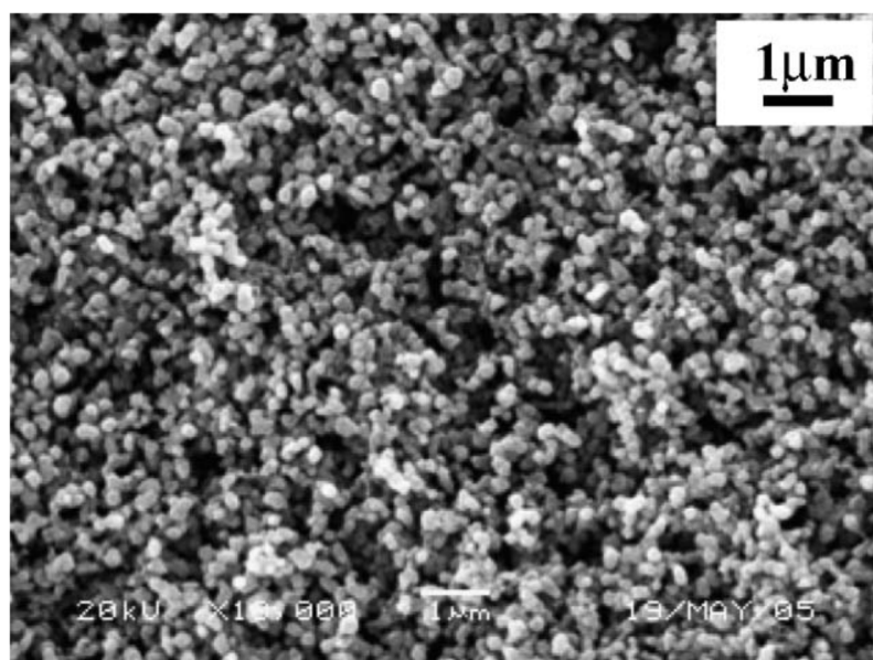
Рис. 11. Микрофотография (СЭМ) порошка NiO, синтезированного термическим разложением смеси ацетата никеля и поливинилацетата [76].
