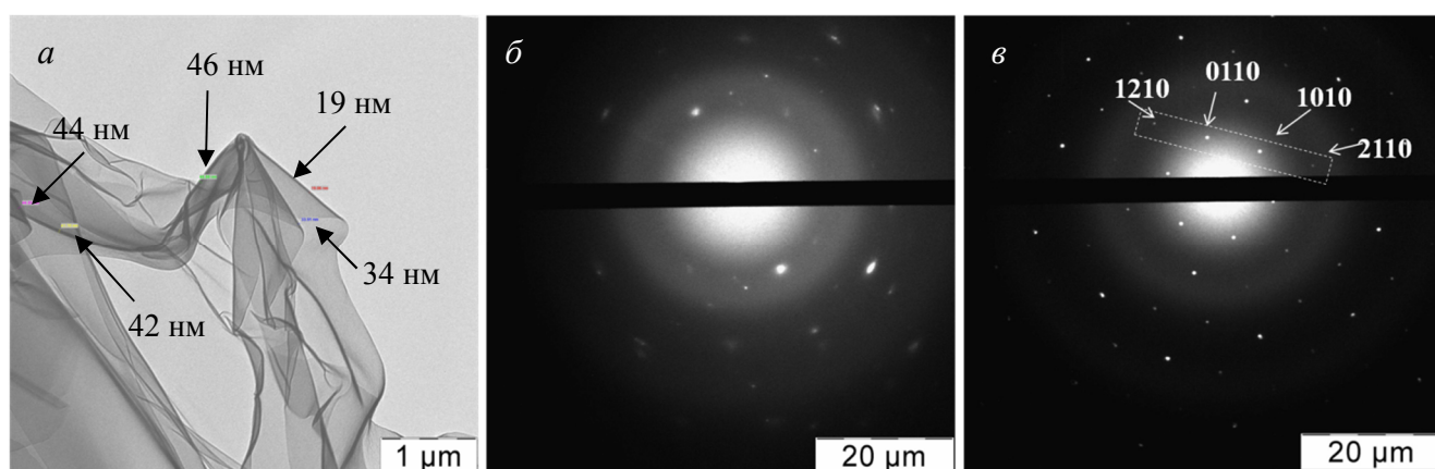
Рис 93. Микрофотография легкой фракции графена, полученная с помощью ПЭМ, (а) и картины дифракция электронов на ней, полученные в разных ее областях (б и в).
