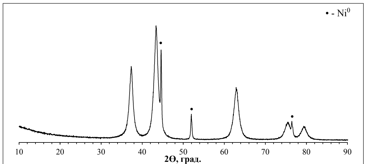
Рис. 129. Дифрактограмма (CuK \alpha ) композита графен-NiO
